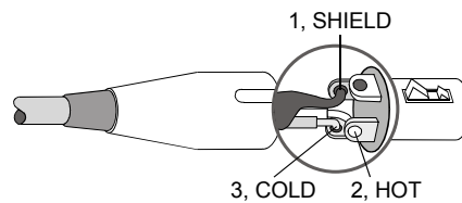
Illustration 2.12 : Connexion symétrisé de la sortie (Daisy-Chain)
