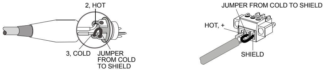
Abbildung 2.11: Unsymmetrische Beschaltung des Eingangs
