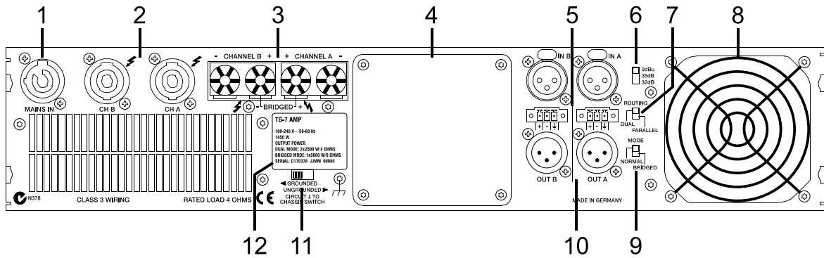
Abbildung 2.2: TG-5/TG-7 Rückseite
