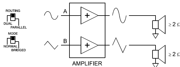
Illustration 2.7 : Signal audio appliqué aux deux connecteurs d'entrée en mode DUAL
