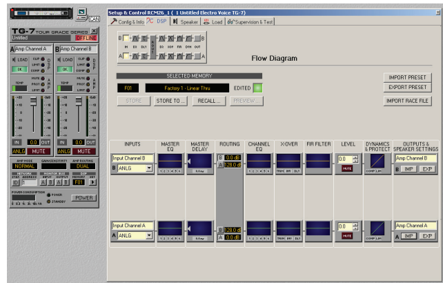
Abbildung 4.3: Bedienpanel und DSP-Flussdiagramm in IRIS-Net™
