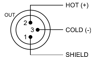
Illustration 4.6: Câblage de la prise AES/EBU-OUT
