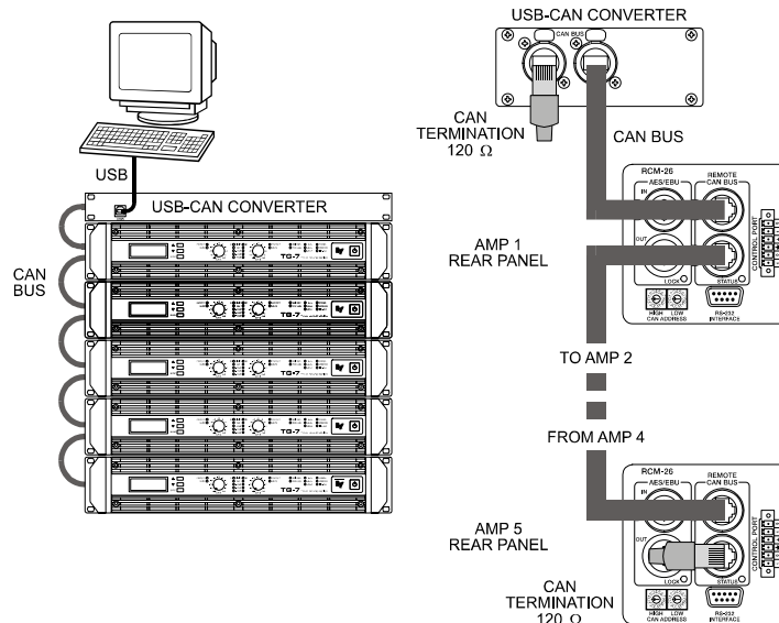
Illustration 4.11: Système avec 5 amplis de puissance et un UCC-1 au début de la chaîne (bus). Bouchons de terminaison sur le UCC-1 (première unité du bus) et sur l'ampli 5 (dernière unité du bus).
