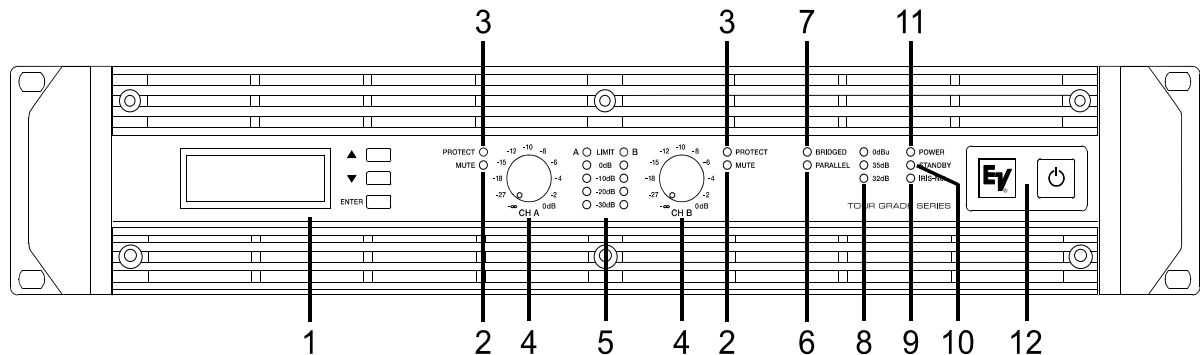
Abbildung 2.1: TG-5/TG-7 Frontseite
