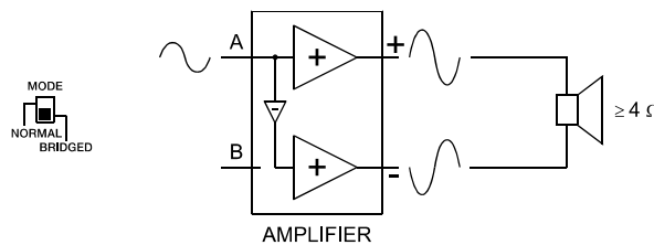
Abbildung 2.9: Betriebsart BRIDGED
