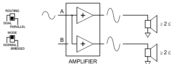
Illustration 2.8 : Signal audio appliqué au connecteur d'entrée A en mode PARALLEL
