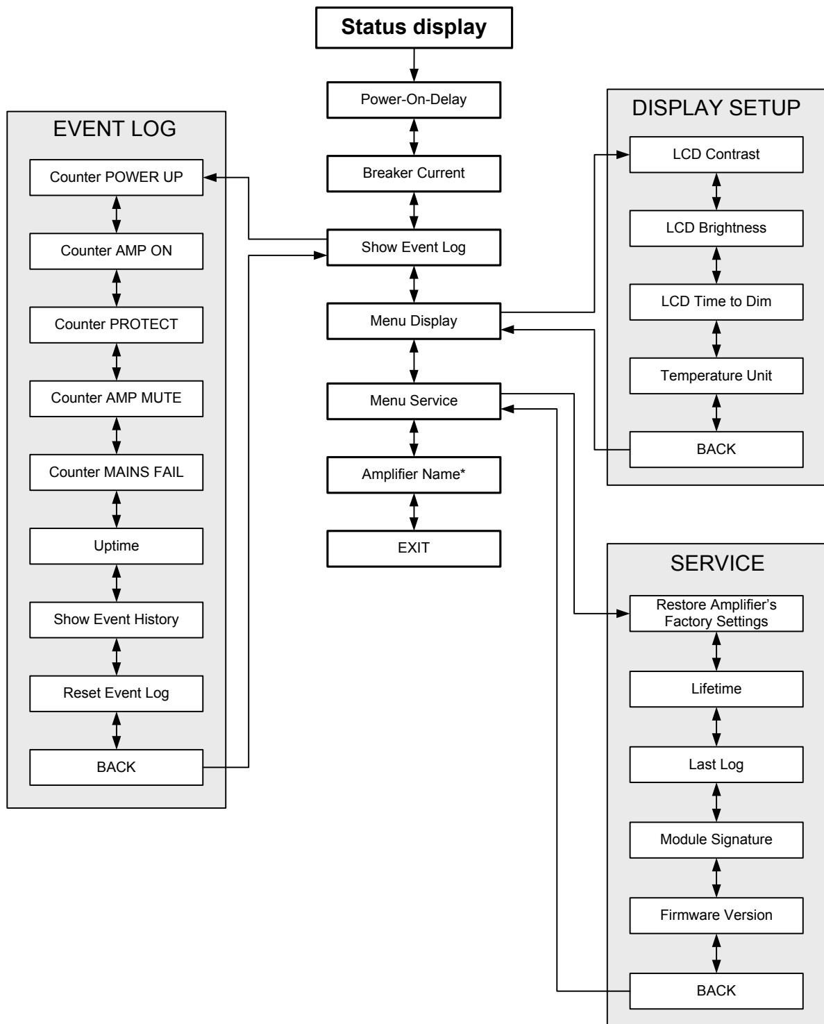
Illustration 3.4 : Structure des menus de l'ampli de puissance
