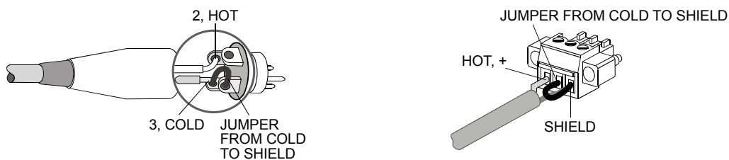
Illustration 2.11 : Connexion non-symétrisée de l'entrée
