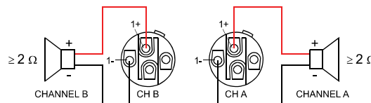
Illustration 2.13 : Connexion de haut-parleur en mode de fonctionnement NORMAL, à l'aide des connecteurs Speakon A et B
