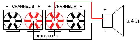
Illustration 2.17 : Connexion de haut-parleur en mode de fonctionnement BRIDGED, à l'aide des bornes
