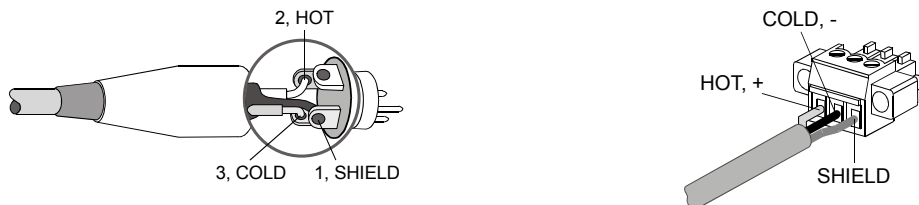
Abbildung 2.10: Symmetrische Beschaltung des Eingangs
