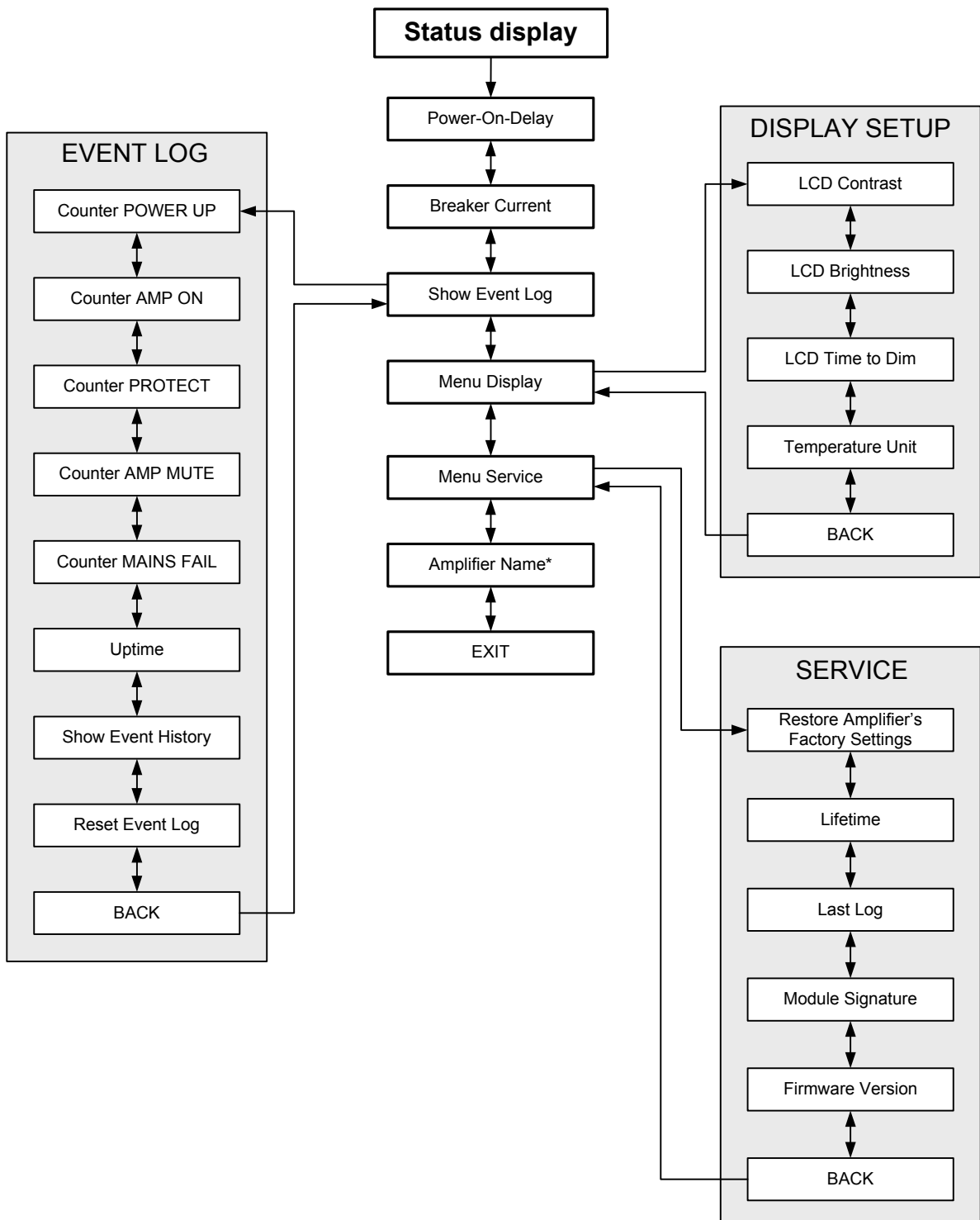
Abbildung 3.4: Menüstruktur der Endstufe
