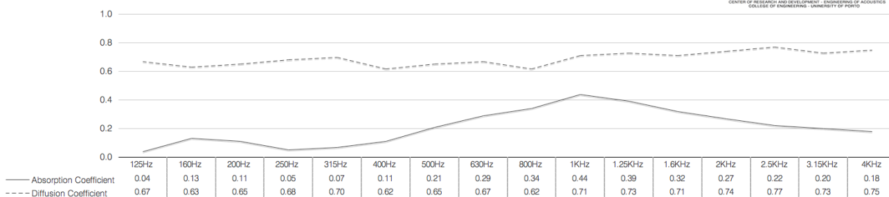
Absorption / Diffusion coefficient - Multifuser DC 2
