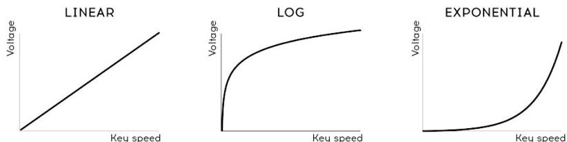
Courbes de vitesse
