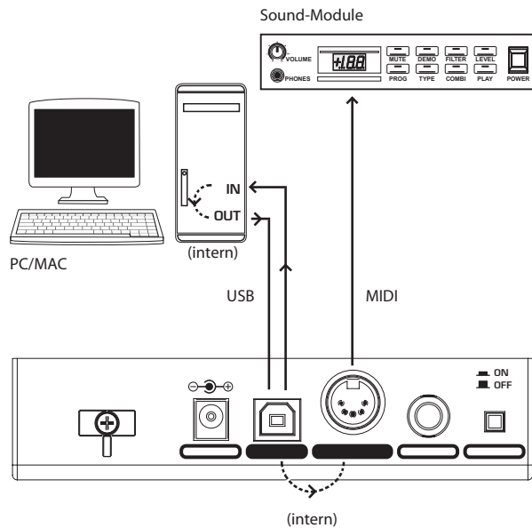
Abb 2.1: Blockschaubild des MIDI-Signalfusses
