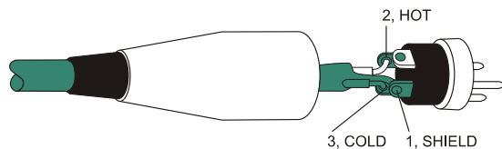
XLR (male)
