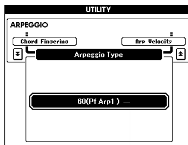
Arpeggio-Typ
